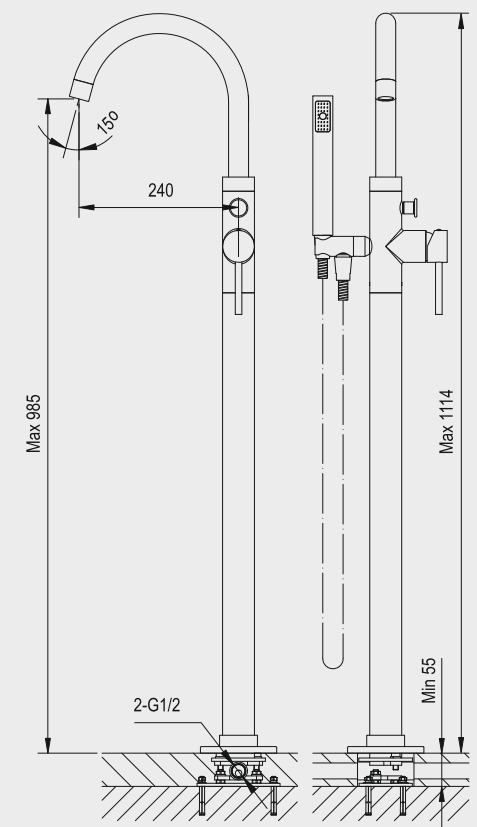
LIVA gold edition Bateria wannowa wolnostojąca
