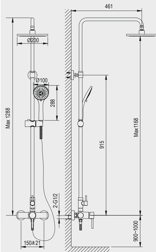
LIVA black edition Zestaw natynkowy natryskowy
