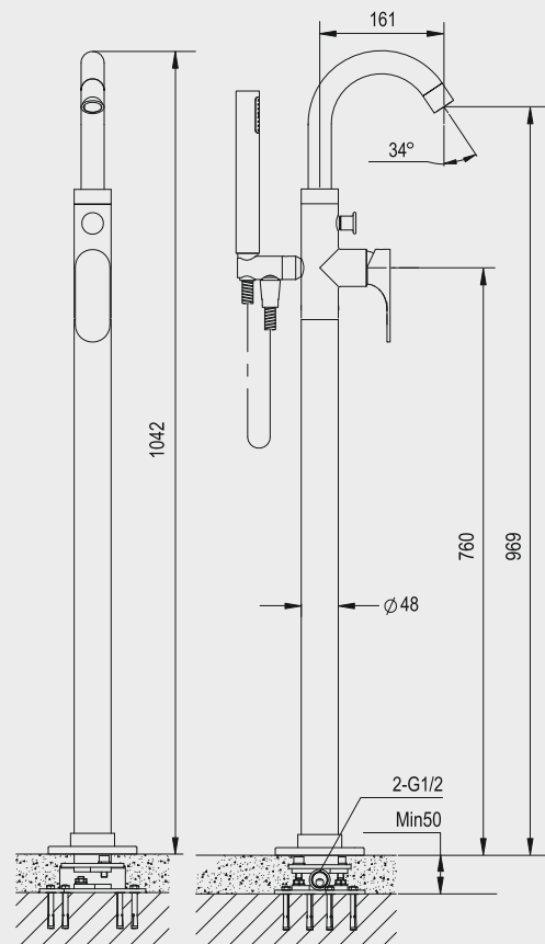
SHENYA chrome Bateria wannowa wolnostojąca
