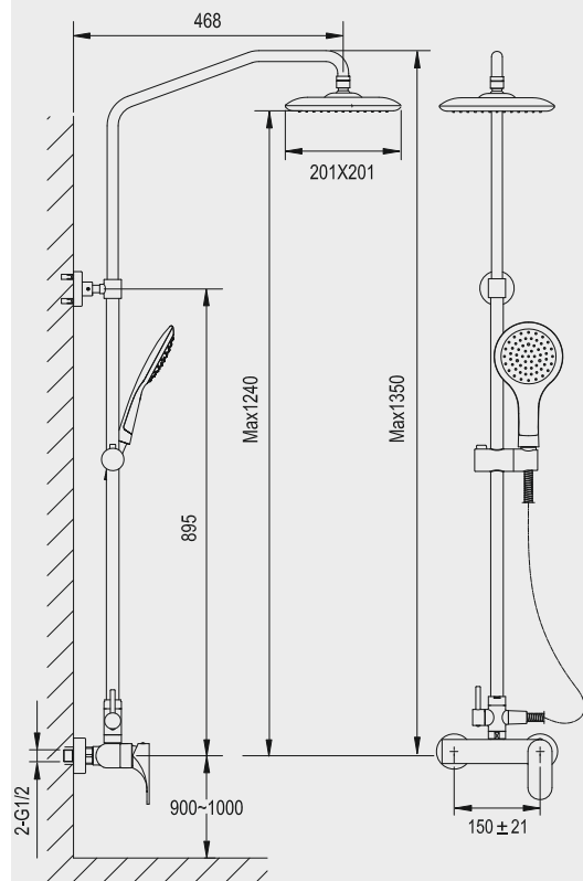
SHENYA chrome Zestaw natryskowy natynkowy
