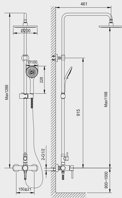
LIVA gold edition Zestaw natryskowy natynkowy
